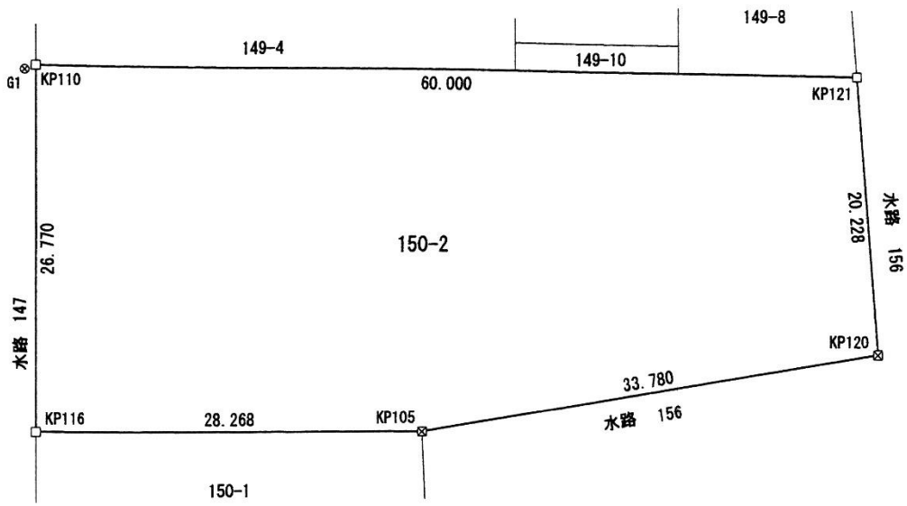
地積測量図
